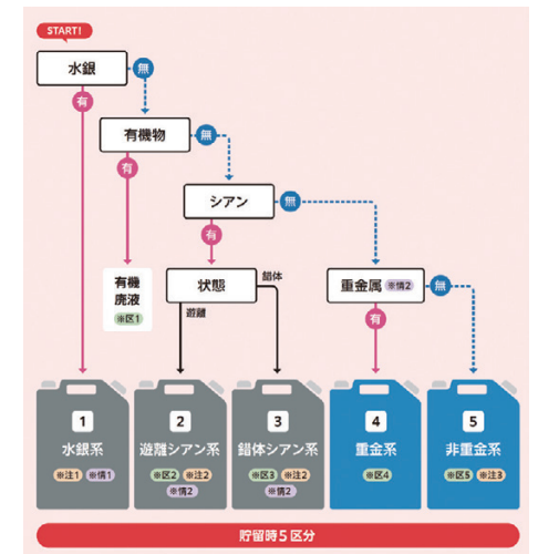
新しい無機廃液の分別貯留チャート
