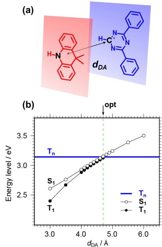
図1 (a) 平行に配したドナーとアクセプターの模式図。(b) (a)におけるドナー/アクセプター距離を変化させた場合の S_1 、 T_1 、 T_n のエネルギー準位。4.7 Å で3つの準位が一致していることがわかる。
