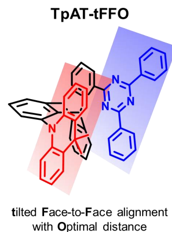
図 2 TpAT-tFFO の構造。ドナーとアクセプターは Face-to-Face の配置から 10^\circ 傾いている。
