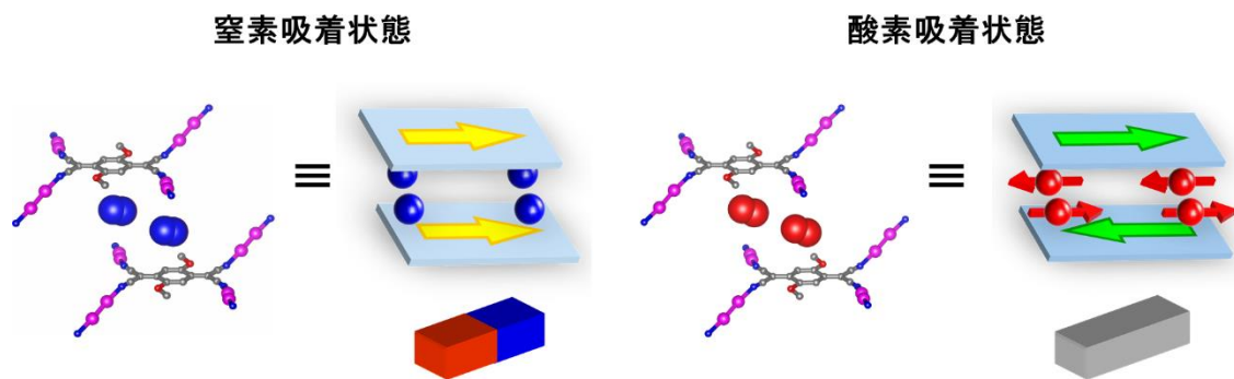
図 5. 窒素吸着型と低圧酸素吸着型の結晶構造（部分：層間に吸着されたガス分子とその周囲骨格のみを示している）とその模式図。どちらも同じ結晶構造であるに関わらず、窒素吸着型は磁石層の磁気モーメント（黄色矢印）同士が平行に配列し、磁石になっており、酸素吸着型は磁石層の磁気モーメント（緑矢印）同士が反平行に配列し打ち消し合い、非磁性となっている。
