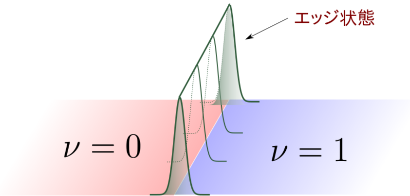
図 1：赤い領域と青い領域は、異なるトポロジカル数 0 と 1 を持つ。そのため、2 つの領域の境界には、接合面に局在した特殊な状態（エッジ状態）が現れる。縦軸は、粒子の存在確率を表す。
