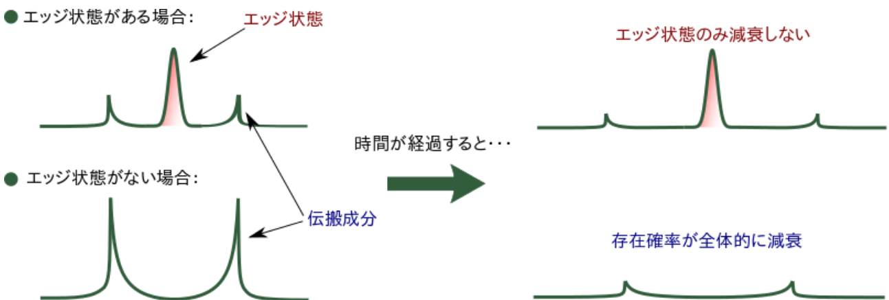
図 2：エッジ状態がある場合（上図）とない場合（下図）における PT 対称な量子ウォークの存在確率とその時間変化。エッジ状態がある場合、図の中央にあるエッジ状態に対応する光子の存在確率は、時間がたっても中央に局在したままで、ほとんど減衰しない。エッジ状態がない場合は、光子の存在確率が全体的に減衰する。
