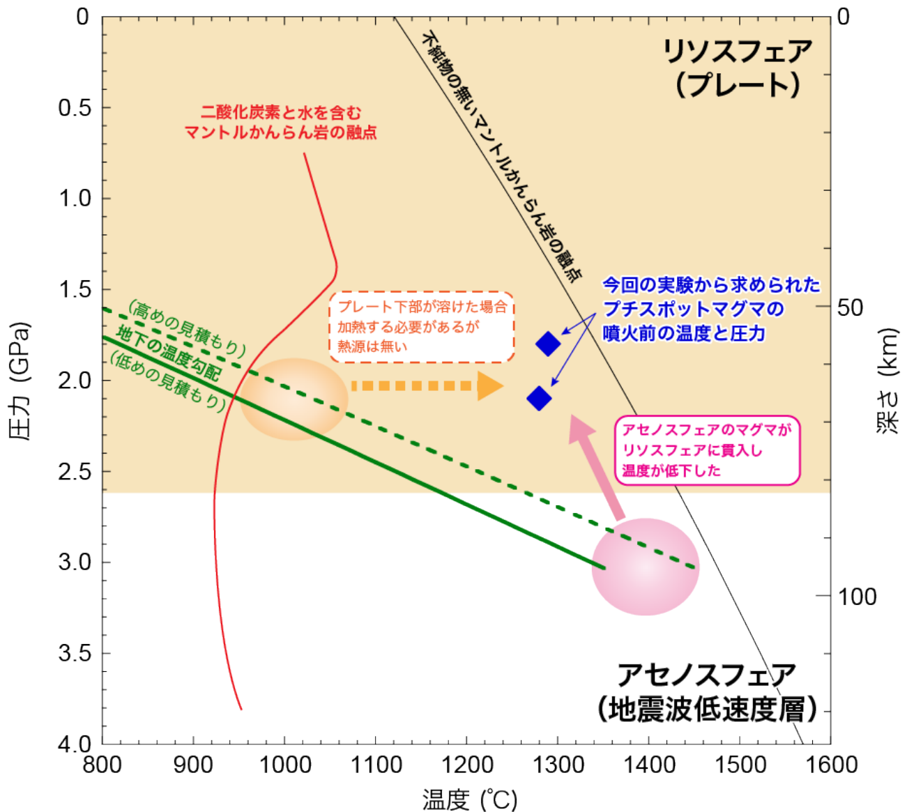
図5：今回の実験から求められたプチスポットマグマの噴火前の最終平衡温度圧力条件と、マンツルかんらん岩の融点および地下の温度勾配とを比較したグラフ（Machida et al. (2017) の Figure 4 を改変・簡略化）。北西太平洋のプチスポット周辺のリソスフェア（プレート）に相当する圧力（厚さ 82 km）を黄色で塗りつぶしている。
