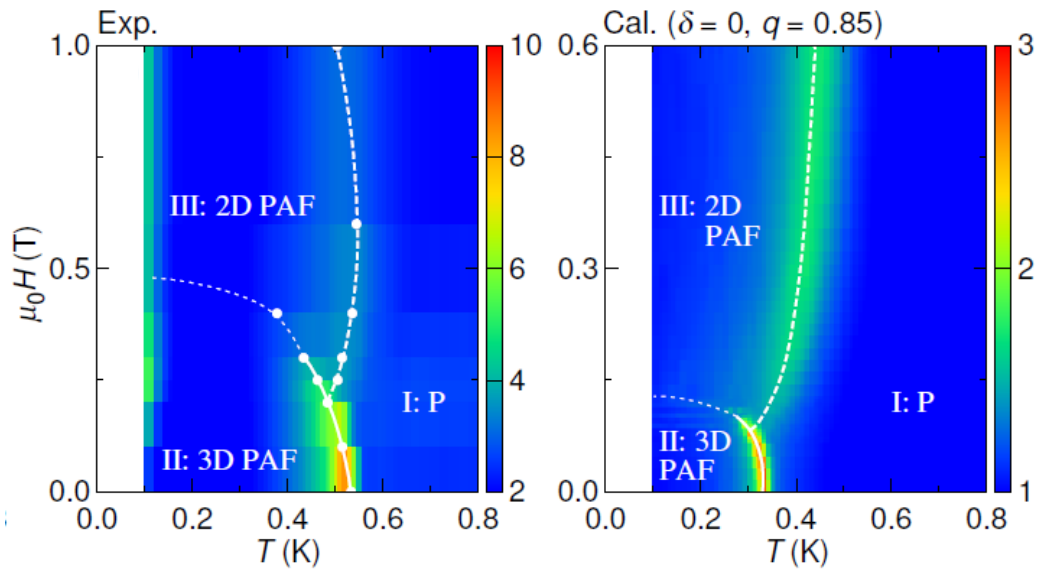
図 3. [111]磁場下の比熱の実験結果(左)と計算結果(右)の比較。量子スピニアイス模型による計算は定性的に実験結果を再現することがわかりました。低磁場領域で温度を下げると高温の常磁性相 (P) から 3 次元の PAF と呼ばれる四極子秩序(3D PAF、図 1 に示した紫丸の秩序構造)の状態になることがわかりました。また、磁場を上げると結晶構造の特徴等を反映して、カゴメ格子面のみで四極子が秩序化する 2 次元の状態 (2D PAF)になることがわかりました。
