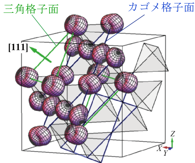
図 1. \text{Tb}_2\text{Ti}_2\text{O}_7 の結晶構造と四極子秩序構造。 \text{Tb}_2\text{Ti}_2\text{O}_7 は、パイロクロア格子と呼ばれる四面体（グレーのピラミッド）が点共有で 3 次的に連なった構造を形成します。四面体頂点にはテルビウムイオンが配置しており、紫色の歪んだ球は四極子秩序後のテルビウムイオンの電荷分布を表しています。それらの周期構造が四極子秩序の構造を表します。[111]方向は三角格子面とカゴメ格子面が交互に積層する 2 次元構造が特徴的な方向です。
