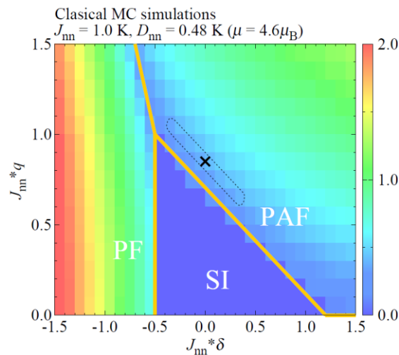
図 4. 古典近似で計算したパラメーター相図。中心のスピニアイス (SI, 量子論的に扱おうと量子スピニアイスになる) の相とそれに隣接して PAF、PF と呼ばれる 2 つの四極子秩序相があります。PAF、PF では四極子の秩序構造が異なります。今回の研究から、実験に見られた \text{Tb}_2\text{Ti}_2\text{O}_7 の秩序は図の点線で囲んだ PAF 領域にあることがわかりました。×印はパラメーターの代表的な一点 (\delta, q) = (0, 0.85) で図 4 右図の計算を行ったパラメーターです。カラー強度は計算から算出された秩序の起きる温度を表しています。
