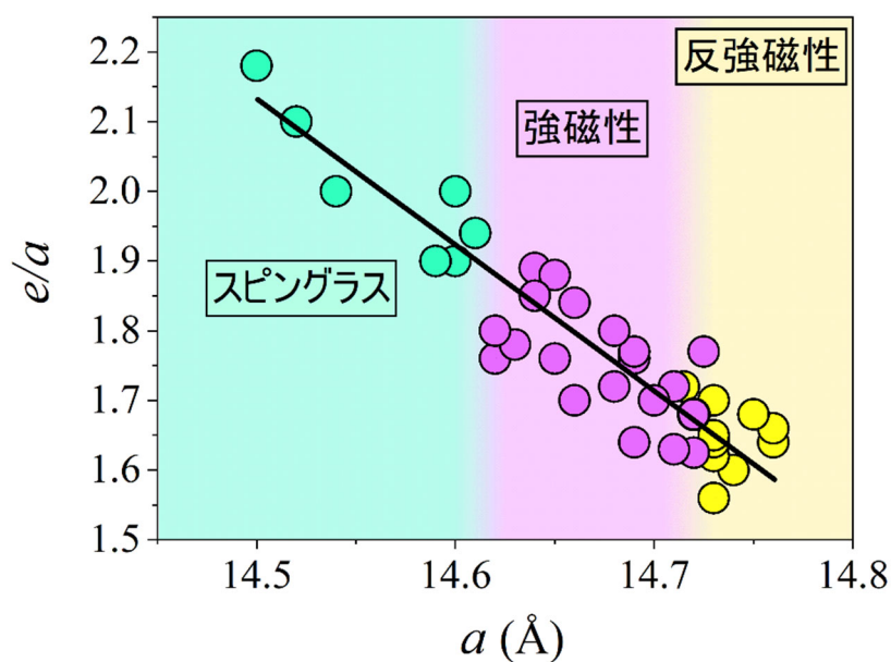
図 3 Tsai 型化合物における磁気相図。Tsai 型化合物の磁気状態を格子定数と価電子濃度 ( e/a ) の関係で整理した結果、スピングラス (Spin-glass)、強磁性 (Ferromagnetic)、反強磁性 (Antiferromagnetic) の各磁気状態が、化学組成や希土類元素の種類によらず、格子定数によって一つの磁気相図上に統一的に分類できることが明らかとなった。従来用いられてきた e/a では物質系によって磁気相境界が異なるのに対し、格子定数を用いると異なる物質系のデータが共通の相境界に集約される。本研究で得られた磁気相図は、新しい磁性準結晶や近似結晶、さらには未知の磁気秩序を示す新物質を探索するための実用的な指針となる。
