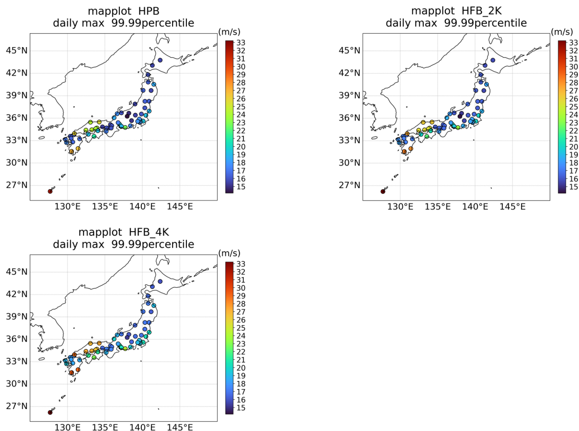
図1 全国主要都市別の日最大風速の気候別の上位 0.01%の極端風速値のマップ。色で風速値を示しています。左上は現在気候、右上は 2°C上昇気候、左下は 4°C上昇気候の場合を示します。
