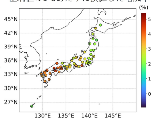
台風時における日最大風速の上位1% 極端値の1°Cあたりに換算した増加率
