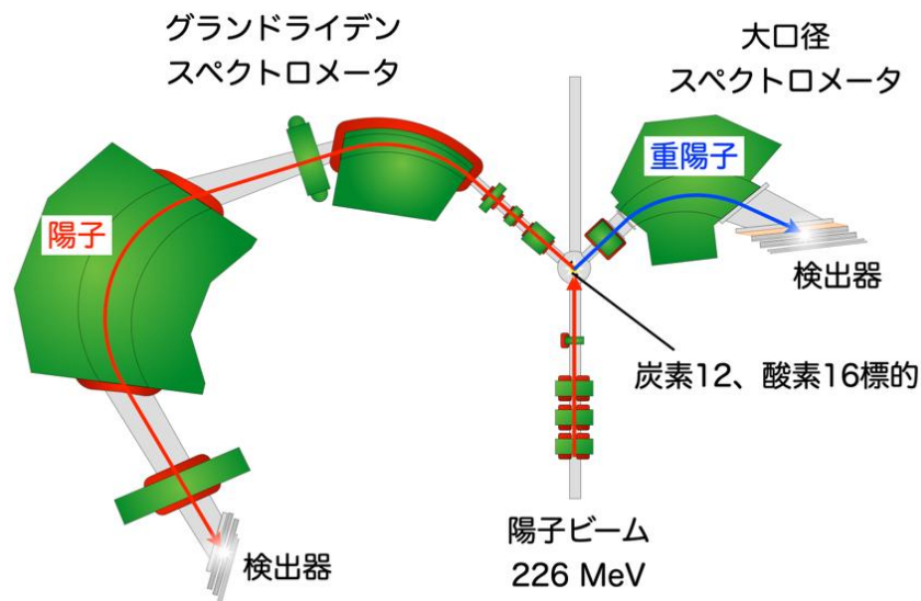
図 3 ノックアウト反応で生じる粒子の分析に用いた装置群
