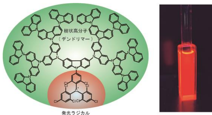
参考図 開発したデンドリマー結合発光ラジカルの構造と発光写真
