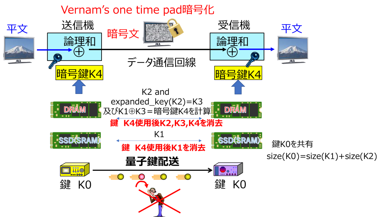
図5 鍵データの安全な消去システム
