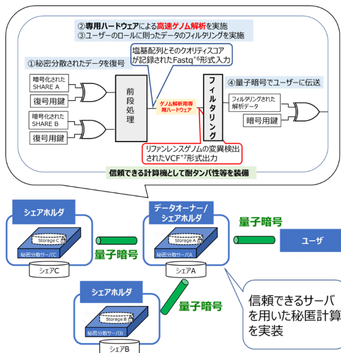
図1 今回開発した“信頼できるサーバ”を実装した量子セキュアクラウド
