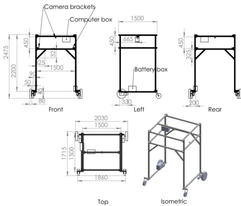
図 3. 今回開発した高速フェノタイピングローバーの 3D 図面。自由に回転や拡大、改変することのできるデータファイルを論文で公開した。
