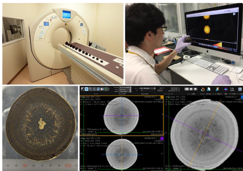
図2. X線CT装置とマンガンノジュールのCTスキャンの例
