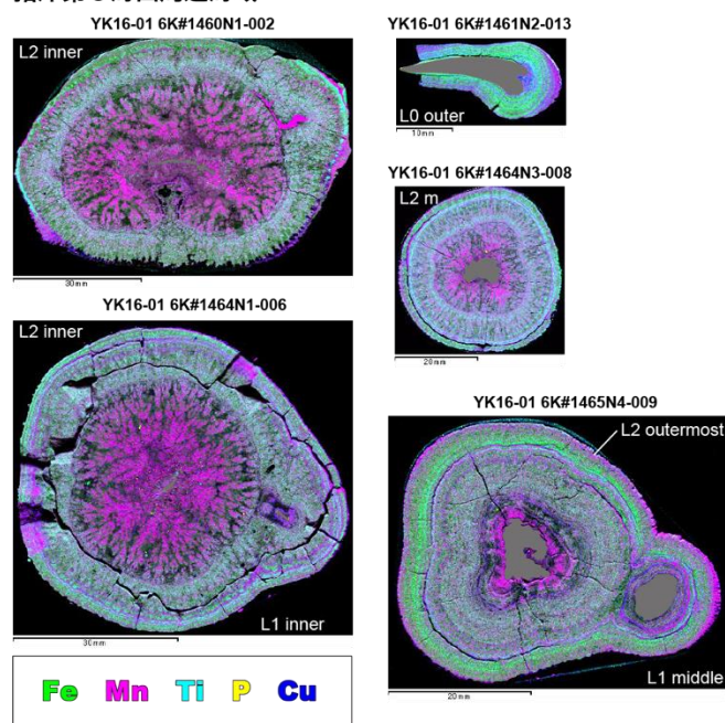
図4. 大きさの異なるマンガンノジュールに対する微小領域蛍光 X 線分析の結果 中心のグレーの部分は核。同定した「最内層」の名前を白字で示している。
