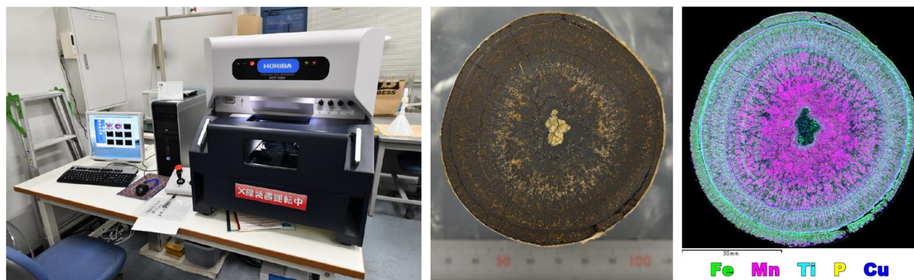
図3. 微小領域蛍光X線分析装置とマンガンノジュールの分析例(図2下に示したものと同一試料)
