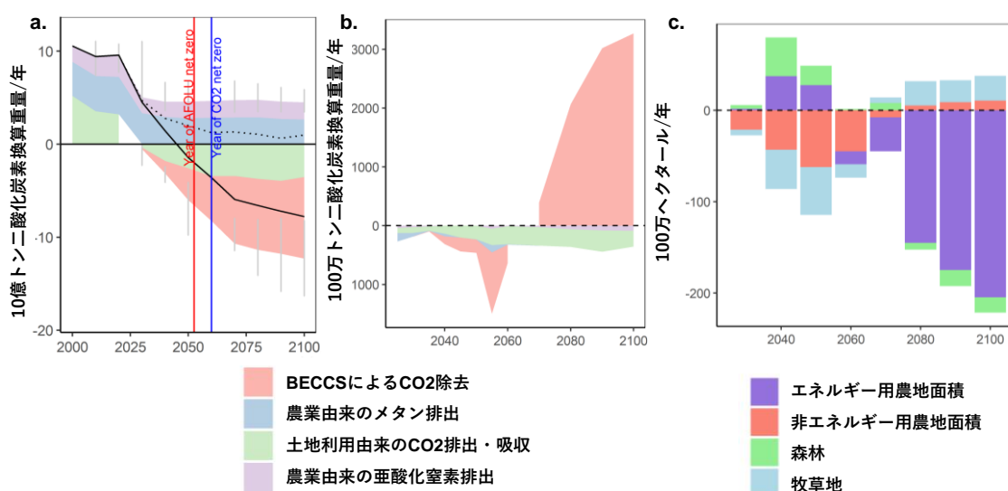
図1 aは大規模な二酸化炭素(CO 2 )除去に依存しないケースの世界全体の農業・土地利用変化由来の温室効果ガス排出経路。b,cは大規模なCO 2 除去技術に依存しないことによる世界全体の農業・土地利用変化由来の温室効果ガス排出と土地利用への影響(大規模なCO 2 除去に依存するケースとしないケースの差分を表す)。aの黒の実線(破線)はBECCS由来のCO 2 除去を含む(含まない)農業・土地利用由来の温室効果ガス(GHG)純排出量を示す。青と赤の縦線は世界全体のCO 2 排出と農業・土地利用由来のGHG排出が実質ゼロに到達する年を示す。土地利用由来のCO 2 排出・吸収には土地利用変化によるCO 2 排出と植林による吸収を含む。
