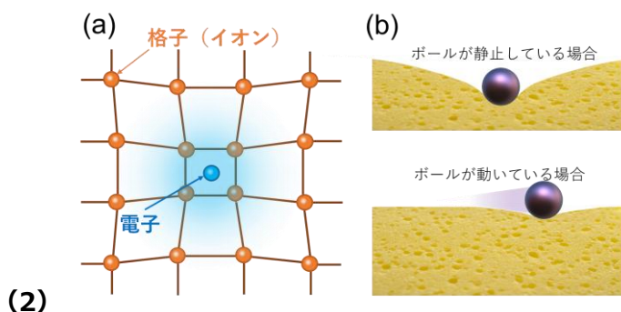
図 2 (a) ポーラロン効果の模式図。電子が周囲の格子（イオンの配置）を歪めて安定化する。(b) スポンジの上に置いたボールの様子。静止したボールは深く沈むが、動いているボールは沈みにくい。
