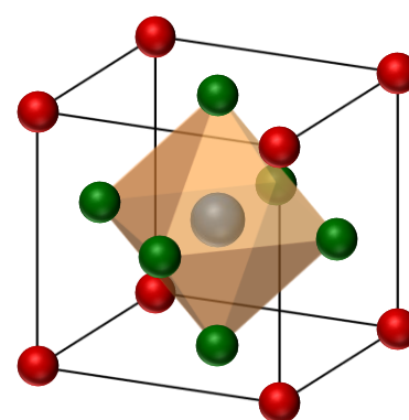
図 1 ABX 3 型ペロブスカイト構造の模式図。立方体の角に A イオン (CH 3 NH 3 , CH 2 (NH 2 ) 2 , Cs など)、中心に B イオン (Pb, Sn)、面心の位置に X イオン (I, Br, Cl) が入る。
