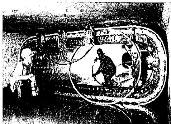
SPR工法によるロサンゼルス下水道管更生工事
