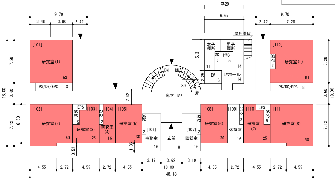
1階平面図 S=1/400
