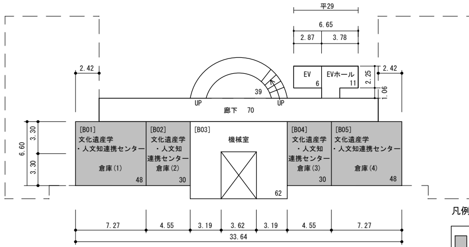
地階平面図 S=1/400
