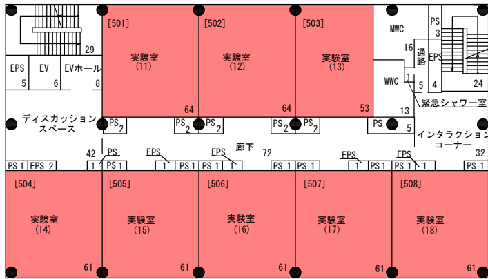
5階平面図 S=1/400
