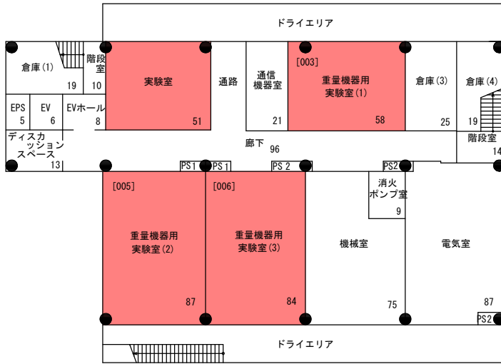
地階平面図 S=1/400
