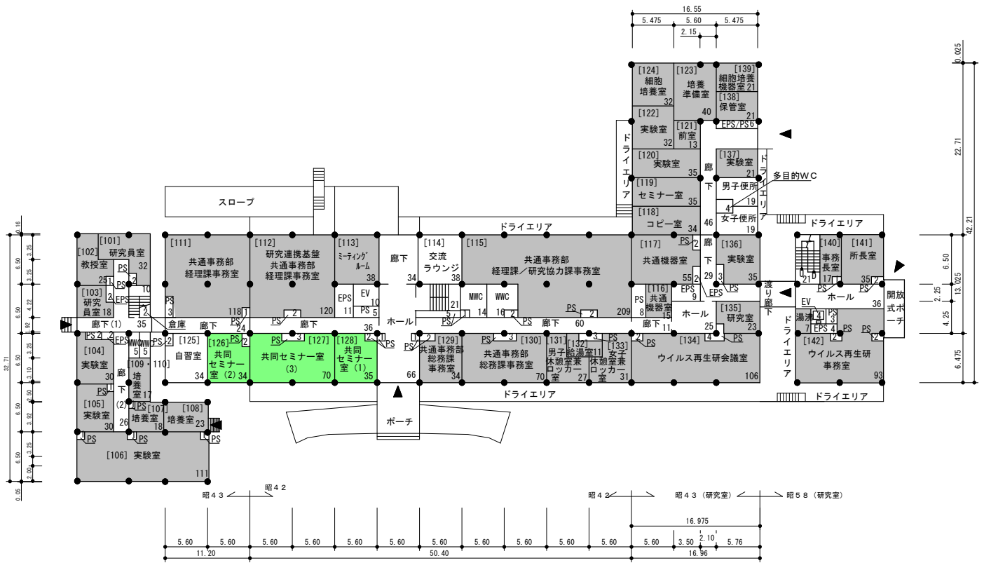
1階平面図 S=1/700
