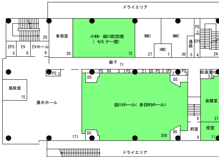
1階平面図 S=1/400
