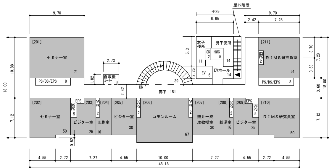
2階平面図 S=1/400
