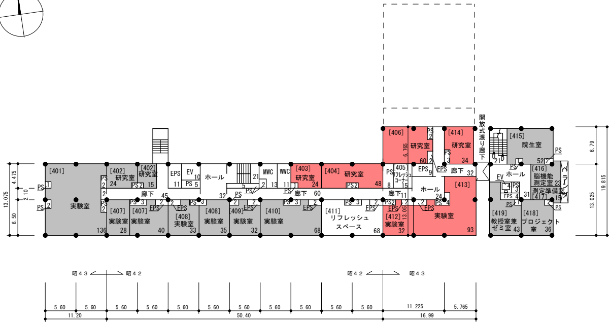
4階平面図 S=1/700
