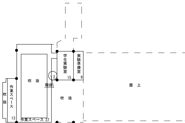
3階平面図 S=1/400
