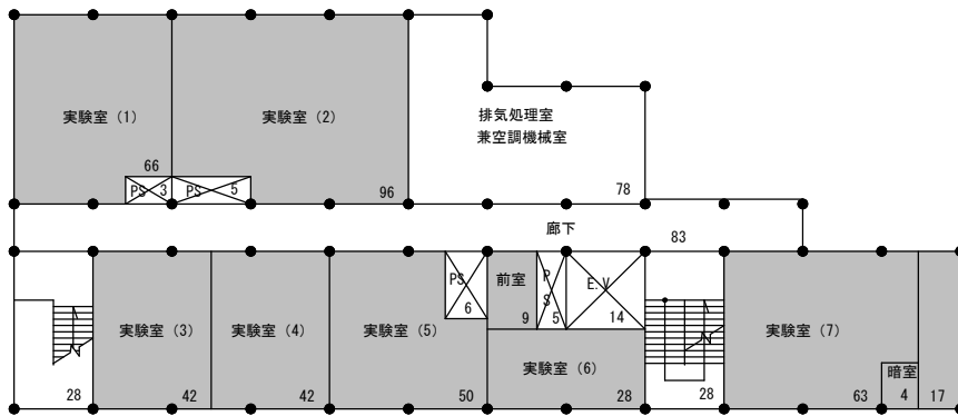
3階平面図 S=1/400
