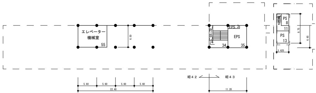
屋階平面図 S=1/700
