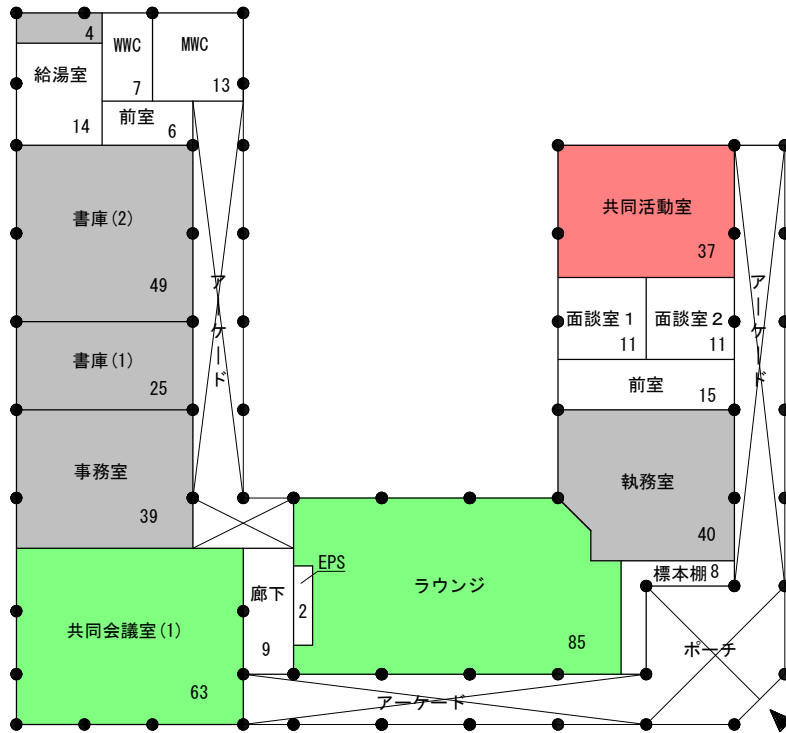
1階平面図 S=1/300
