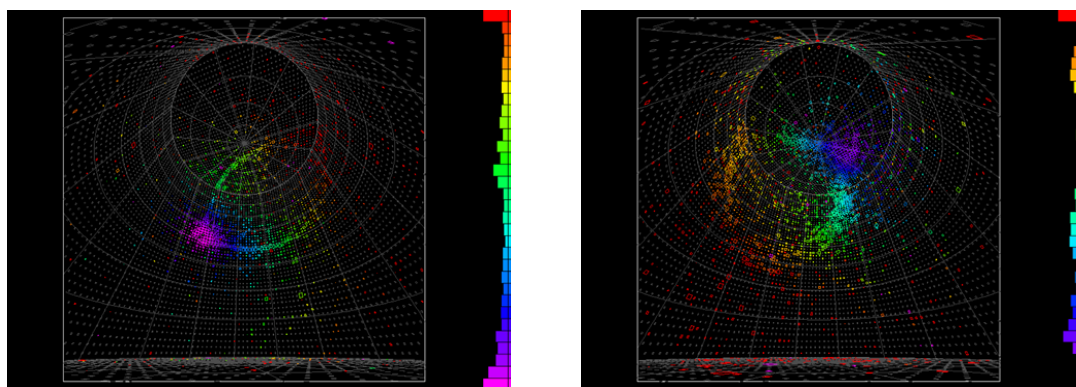
図 2 : スーパーカミオカンデで検出された電子型のニュートリノ (左) と反ニュートリノ (右) の例。ニュートリノが水と反応してできた電子、または陽電子によるリング状の微弱光を、タンク内壁に設置された約 11000 本の光電子増倍管で観測しています。色のついた点は、その光電子増倍管で光を検出した時間を表しています。
