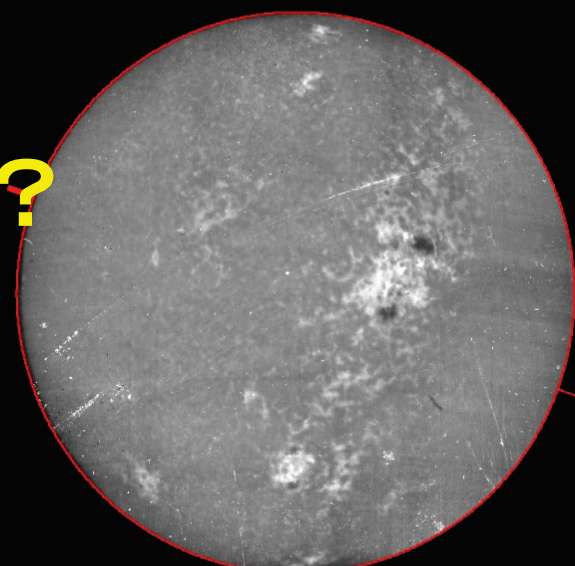
太陽全面カルシウムK線画像(京大生駒山太陽観測所)
